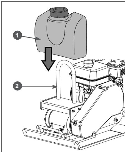
Рис. 19 Установка бака
