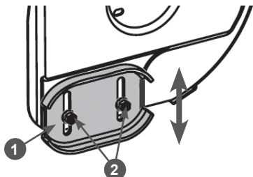
Рис. 29 Регулировка высоты забора снега 1. Ползков 2. Гайка (2 шт.)
