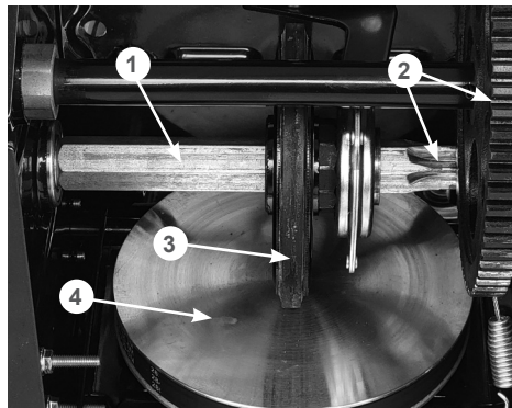
Рис. 46 Обслуживание трансмиссии
