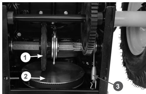
Рис. 12 Регулировка троса включения хода
