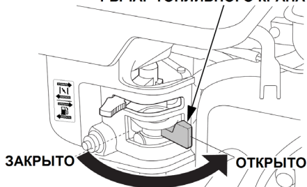
Рис. 31 Рычаг топливного крана
