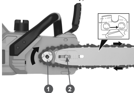
Рис. 3. Установка цепи
