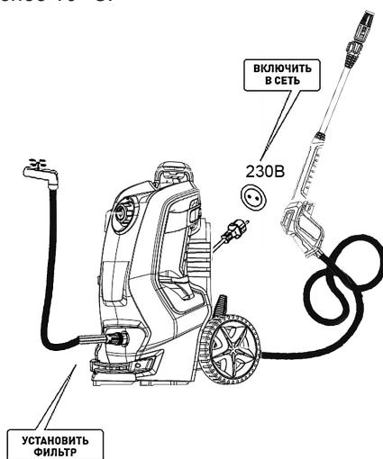
Рис. 6 Подключение аппарата высокого давления
