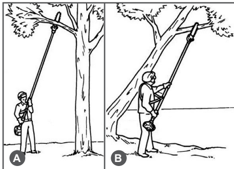
Рис. 17. Положение оператора при работе
