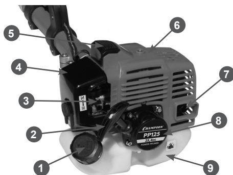
Рис. 4. Основные узлы и органы управления (двигатель)
