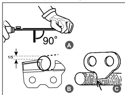
Рис. 28. Положение напильника при заточке
