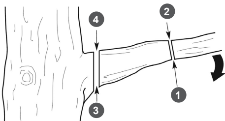
Рис. 19. Последовательность резов при отпиливании толстых веток
