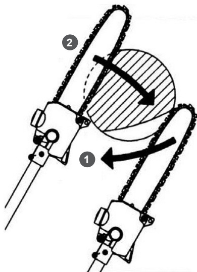
Рис. 18. Выполнение разгрузочного и основного резов
