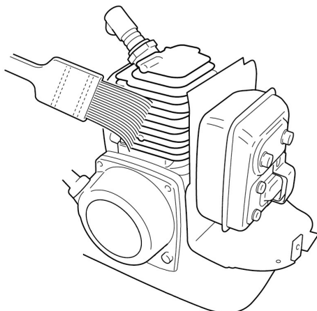
Рис. 22. Очистка рёбер охлаждения цилиндра
