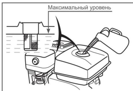
Рис. 10 Максимальный уровень топлива в топливном баке
