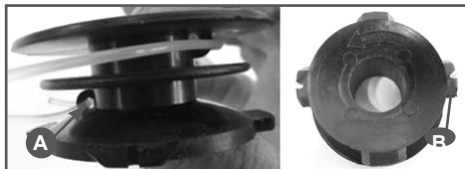
Рис. 24 Установка корда
