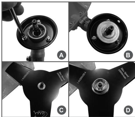
Рис. 4 Установка ножа
