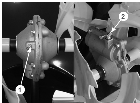
Рис. 43 Добавление смазки в редуктор
