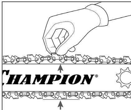
Рис. 8 Положение цепи на шине
