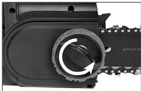
Рис. 4 Откручивание гайки крепления крышки шины
