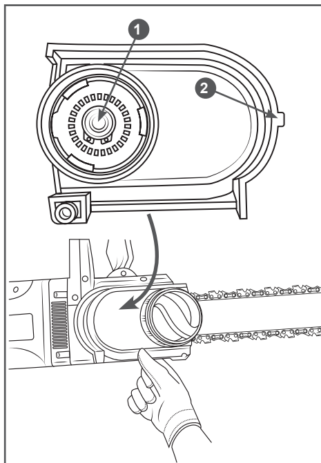
Рис. 6 Установка крышки шины
