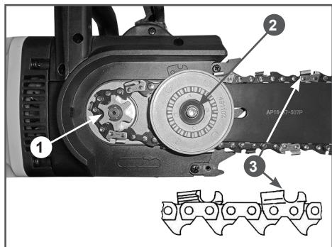
Рис. 5 Установка цепи
