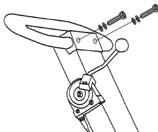
Рис. 3 Установка рабочей рукоятки
