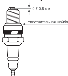
Рис. 19 Обслуживание свечи зажигания
