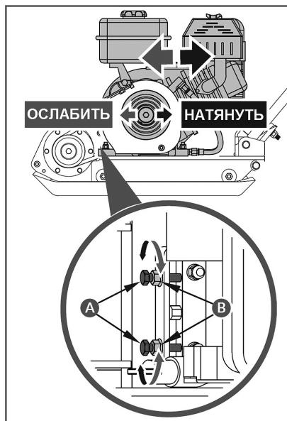
Рис. 26 Регулировка натяжения ремней А – болт В - контргайка
