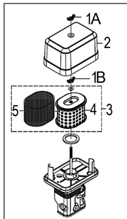
Рис. 17 Обслуживание воздушного фильтра
