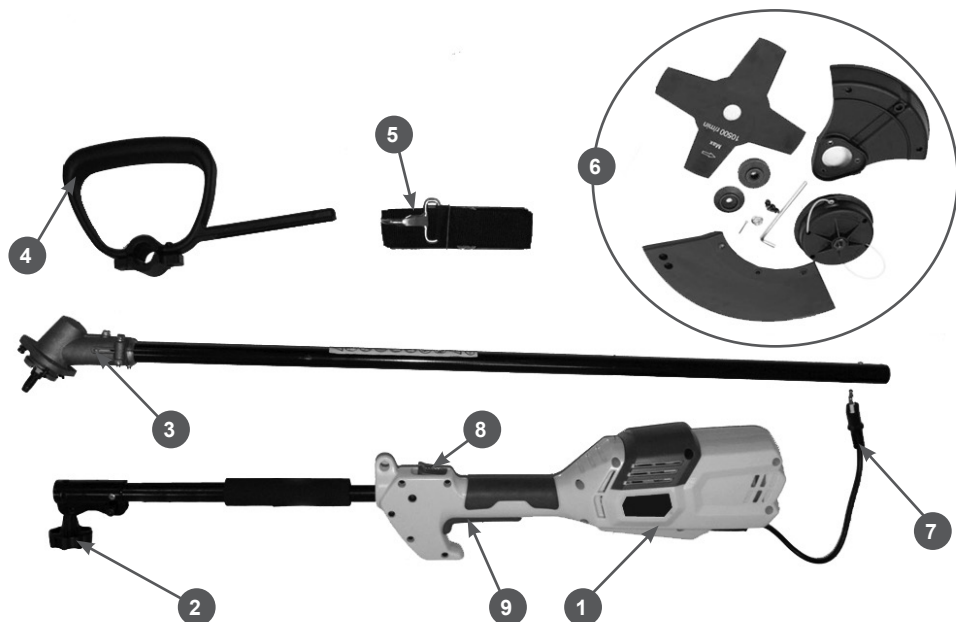
Рис.1 Основные узлы и органы управления
