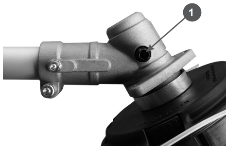
Рис. 20 Болт отверстия для смазки редуктора
