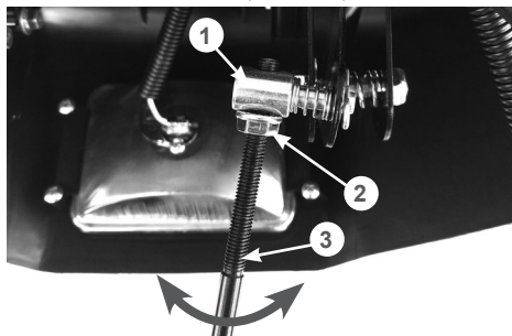
Рис. 17 Регулировка длины туги рычага переключения передач
