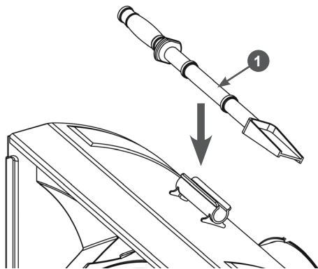
Рис. 36 Расположение лопатки для очистки
