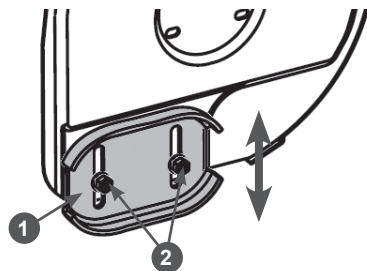
Рис. 29 Регулировка высоты забора снега 1. Полозья 2. Гайка (2 шт.)
