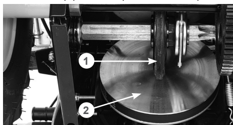
Рис. 16 Проверка нейтрального положения фрикционного колеса
