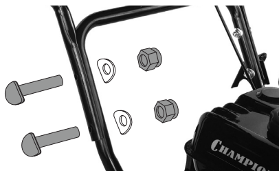
Рис. 5 Установка рукояток
