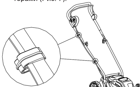
Рис. 7 Установка фиксаторов кабеля включения
