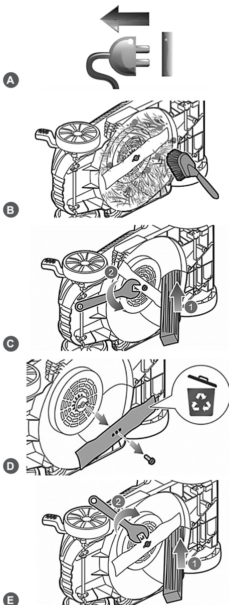
Рис. 18 Замена ножа
