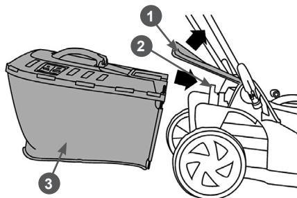
Рис. 6 Установка травосборника 1. Крышка задняя 2. Выступ 3. Травосборник
