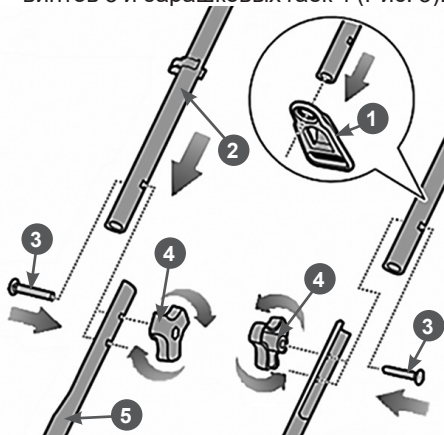
Рис. 3 Сборка рабочей рукоятки
