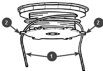
Рис. 14. Фиксация концов корда 1. Концы корда 2. Пазы на катушке
