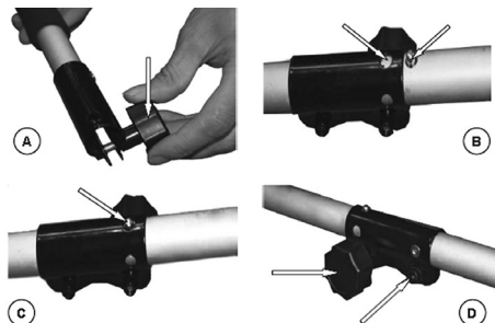
Рис. 5. Установка нижней штанги
