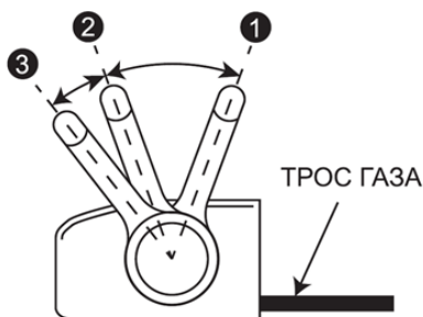
Рис. 15 Положения рычага газа
