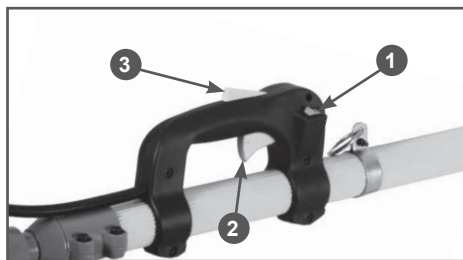
Рис. 9 Органы управления на рабочей рукоятке
