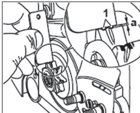
Рис. 21 Обслуживание ведущей звездочки
