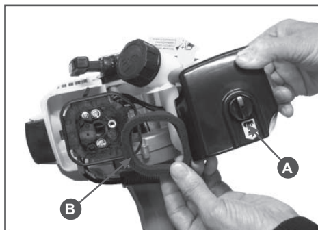
Рис. 13 Обслуживание воздушного фильтра
