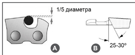
Рис. 19 Положение напильника при заточке режущего зуба
