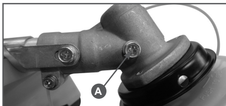
Рис. 17 Обслуживание редуктора
