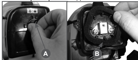
Рис.15 Обслуживание воздушного фильтра
