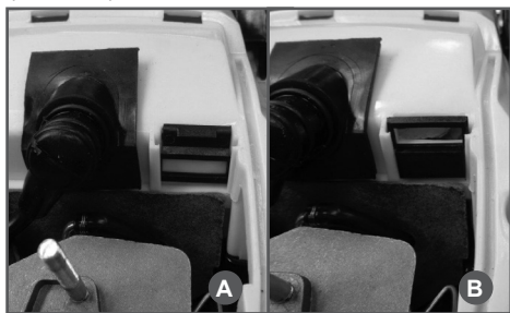
Рис. 9 Положение заглушки «зима-лето»
