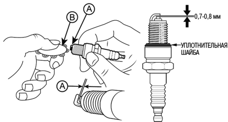
Рис. 12. Проверка зазора между электродами
