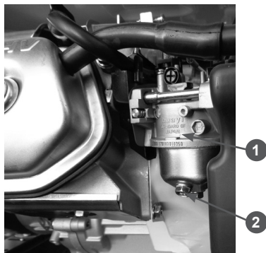
Рис. 10. Слив топлива из карбюратора
