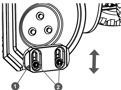
Рис. 20 Регулировка высоты забора снега 1. Полозок 2. Гайка (2 шт.)
