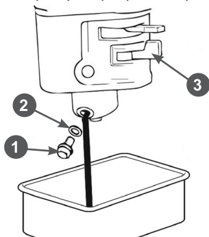
Рис. 31 Обслуживание фильтра-отстойника
