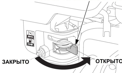
Рис. 22 Рычаг топливного крана
