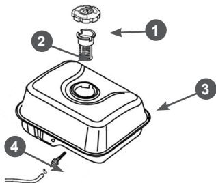
Рис. 29 Топливные фильтры
