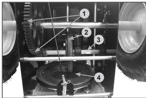
Рис. 35 Обслуживание трансмиссии
