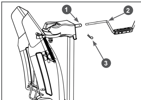
Рис. 16 Крепление вала управления поворотом желоба
