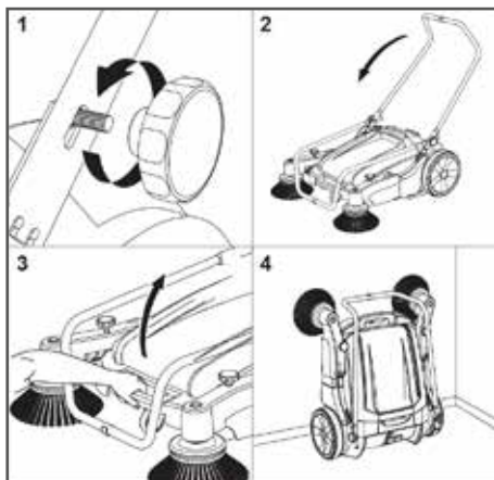
Рис. 17 Хранение машины
