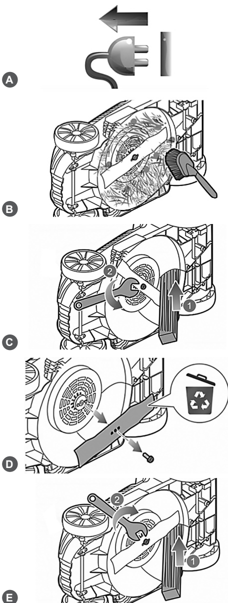
Рис. 18 Замена ножа
