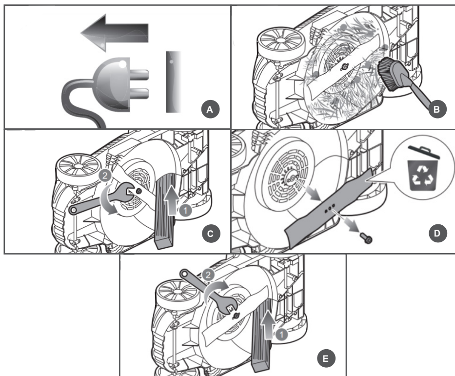
Рис. 15 Снятие-установка ножа
