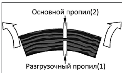
Рис. 16 Распиливание дерева, когда его верхняя часть находится под напряжением
