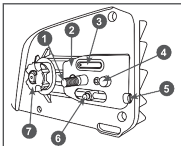
Рис. 3 Снятие крышки шины
