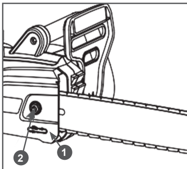
Рис. 2 Снятие крышки шины
