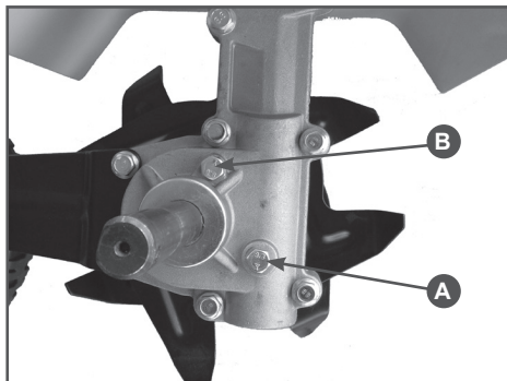
Рис. 23 Обслуживание редуктора
