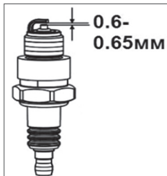
Рис. 22 Свеча зажигания
