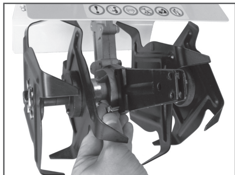
Рис. 5 Установка кронштейна сошника
