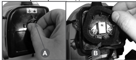
Рис.15 Обслуживание воздушного фильтра
