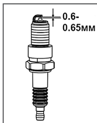
Рис. 16 Определение зазора свечи
