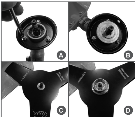
Рис.5 Установка ножа для травы
