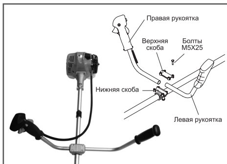
Рис.4 Установка рукояток
