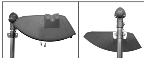
Рис.2 Установка защитного кожуха
