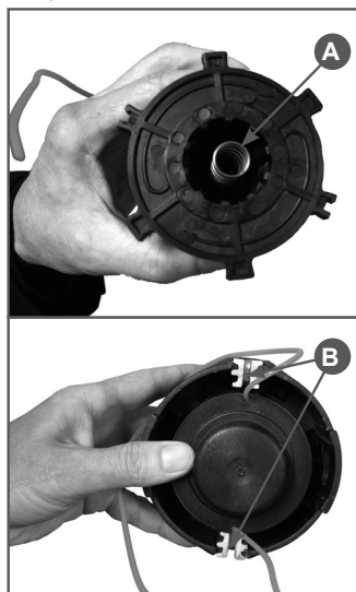
Рис. 19 Установка катушки в корпус
