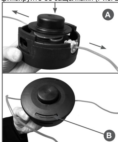
Рис. 20 Сборка триммерной головки
