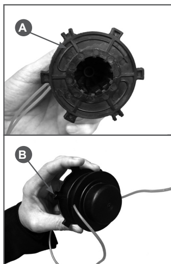
Рис. 18 Намотка корда
