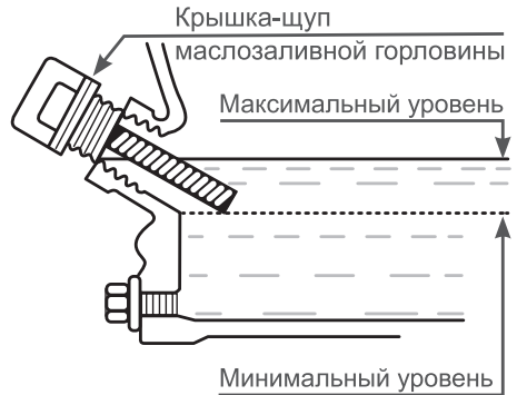
Рис. 5 Проверка уровня масла в картере
