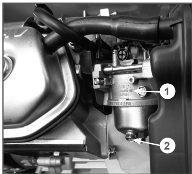
Рис. 20 Слив топлива из карбюратора
