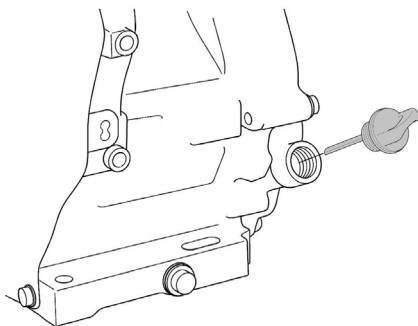
Рис. 8 Крышка-щуп маслосливной горловины
