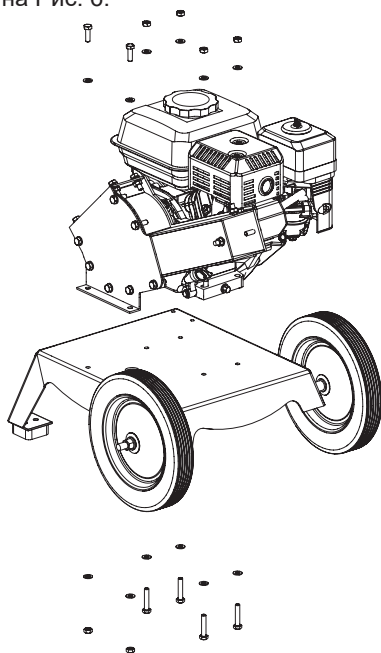
Рис. 6 Схема установки двигателя
