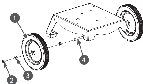
Рис. 5 Схема установка колёс
