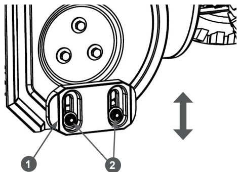
Рис. 17 Регулировка высоты забора снега 1. Полозок 2. Гайка (2 шт.)
