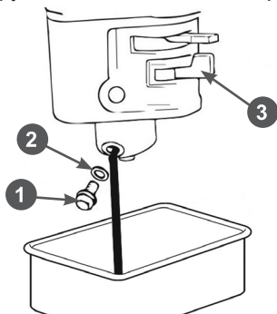
Рис.28 Обслуживание фильтра-отстойника
