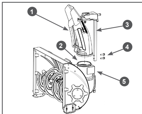
Рис. 10 Установка желоба выброса снега
