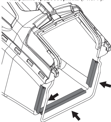
Рис. 7 Крепление нижней части травосборника
