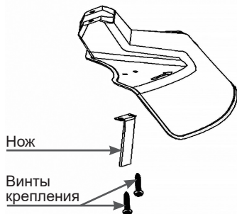
Рис. 2 Установка ножа для обрезки корда
