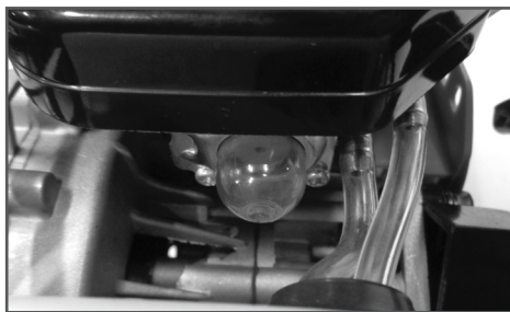
Рис.8 Ручной топливный насос
