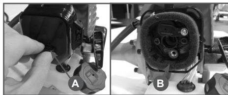
Рис.12 Обслуживание воздушного фильтра
