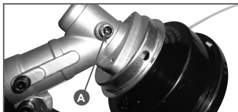
Рис. 14 Обслуживание редуктора
