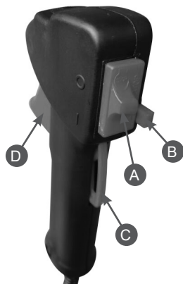
Рис. 9 Рукоятка управления
