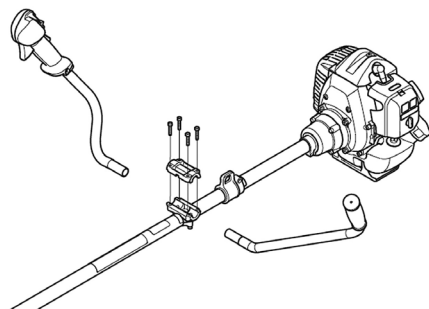
Рис. 6 Установка рукояток
