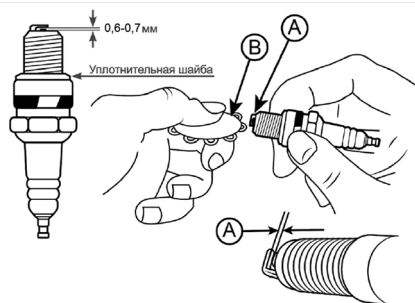
Рис. 15 Проверка зазора между электродами
