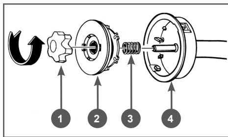
Рис. 9 Снятие триммерной головки
