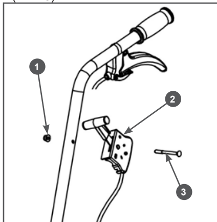
Рис. 8 Установка рычага газа
