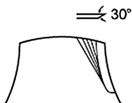
Рис. 16 Заточка ножа
