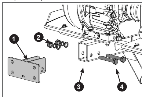
Рис. 12. Установка основания кронштейна для навесной роторной косилки
