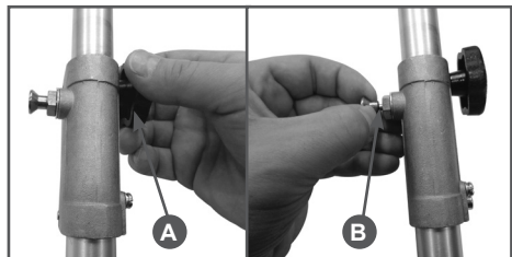
Рис.3 Сборка штанги (для моделей с разъёмной штангой)
