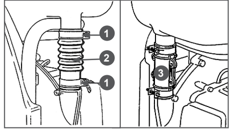
Рис. 12 Замена гибкого шланга подачи воздуха на кожух
